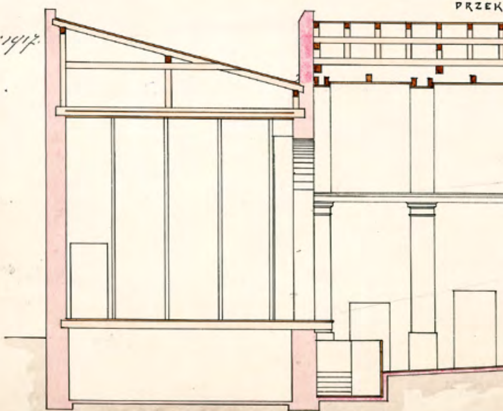
■ Plan kina „Czary”, 1917 r. Starostwo Powiatowe Piotrkowskie, sygn. 138.
