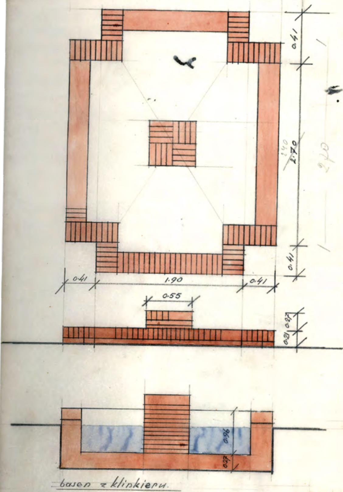
■ Projekt basenu w ogrodzie botanicznym w Piotrkowie, 1933 r. Akta miasta Piotrkowa, sygn. 1905. ■ Project of the swimming pool in the botanic garden in Piotrków, 1933. Records of the city of Piotrków, sig. 1905.
