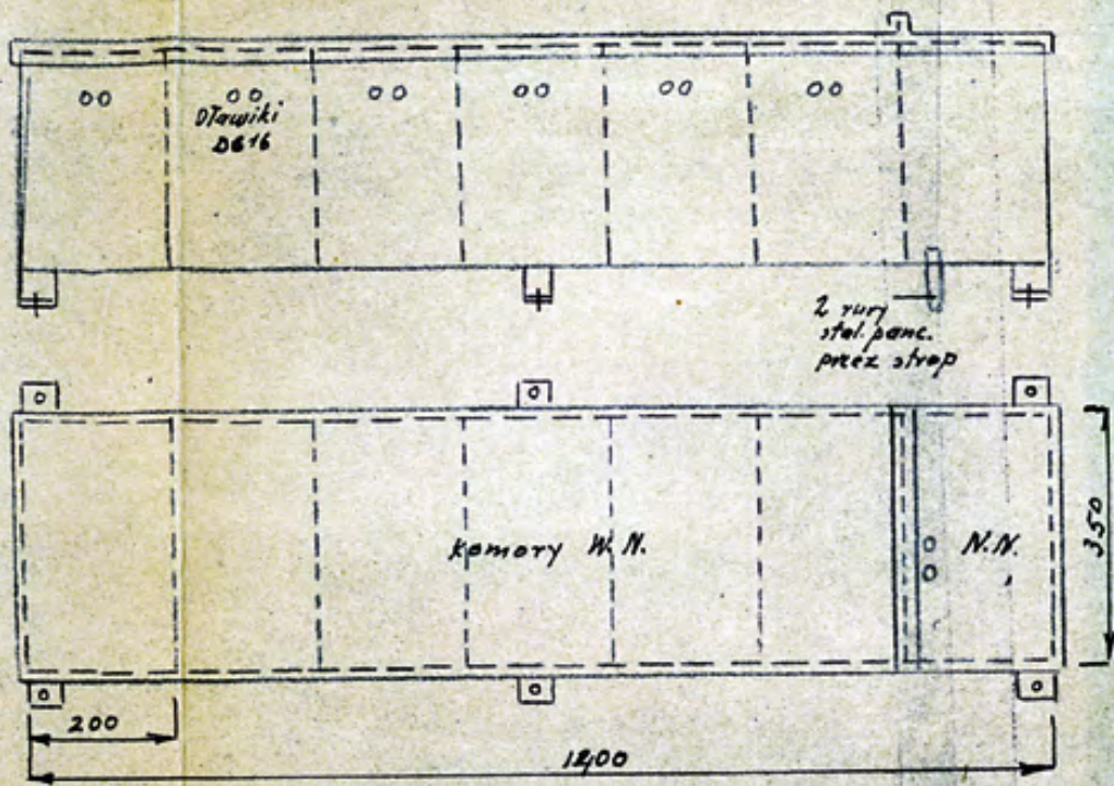
Szkic skrzynki transf. dachowej skala 1:10
