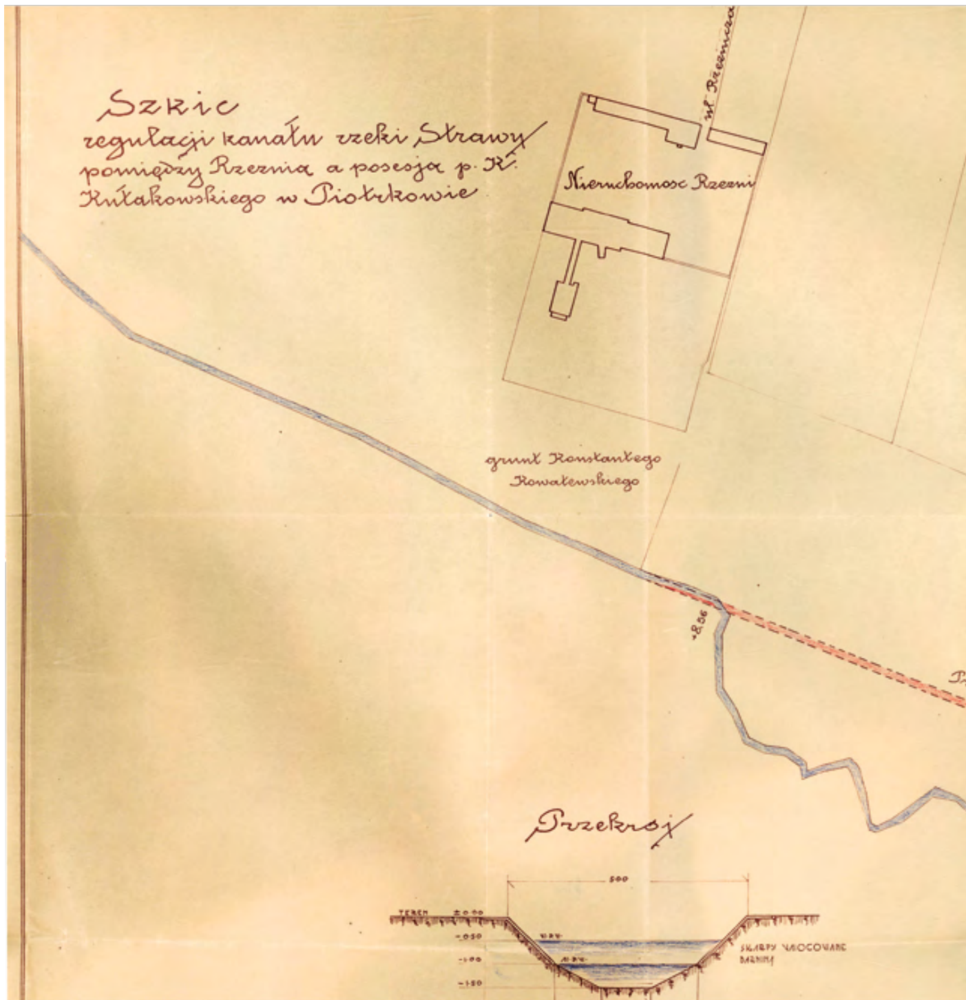
■ Szkic regulacji kanału rz. Strawy, 1933 r. Akta miasta Piotrkowa, sygn. 1893.
